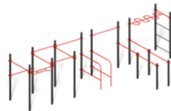
CO-243 Воркаут-комплекс 'Баланс' Д 9450 / Ш 4050 / В 2295 мм
