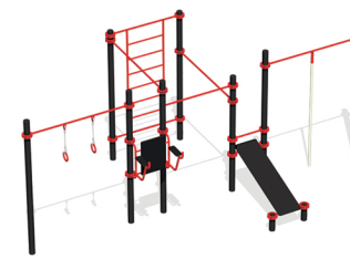
CO-222.1 Снаряд Д 6300 / Ш 3295 / В 2600 мм
