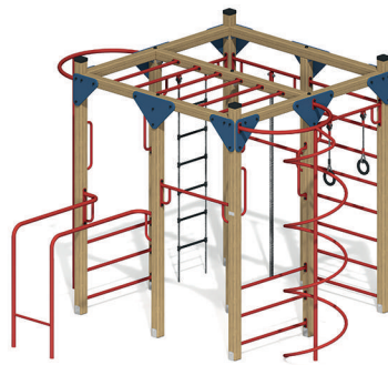
ГК-24 Гимнастический комплекс Д 3810 / Ш 3580 / В 2805 мм
