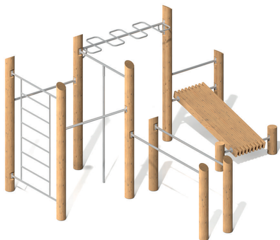
CO-111 Спортивный комплекс Д 5060 / Ш 4265 / В 2770 мм
