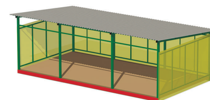
ТН-03 Веранда Д 7830 / Ш 4550 / В 2695 мм
