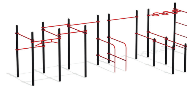
CO-243 Снаряд Д 9110 / Ш 3850 / В 2405 мм
