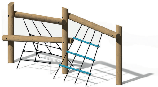
СО-127 Спортивное оборудование "Конструкция для лазания 2" Д 4280 / Ш 1800 / В 2020 мм
