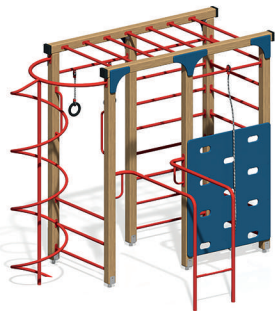
ГК-24М Гимнастический комплекс Д 3240 / Ш 2480 / В 2655 мм
