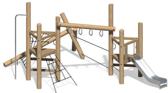
ИК-213 Игровой комплекс Д 7590 / Ш 6190 / В 3600 мм
