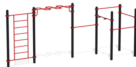
CO-204 Снаряд Д 6080 / Ш 1540 / В 2600 мм
