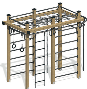
ГК-10.3 Гимнастический комплекс Д 3120 / Ш 1785 / В 2555 мм
