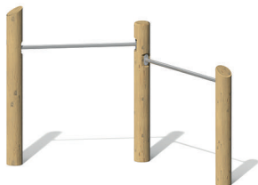
CO-124 Спортивное оборудование "Двойной турник" Д 2240 / Ш 720 / В 1500 мм
