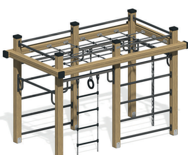
ГК-10.1 Гимнастический комплекс Д 2670 / Ш 1530 / В 1905 мм
