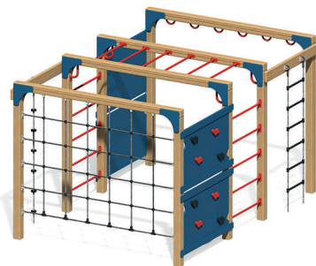
ГК-01.2 Гимнастический комплекс Д 3570 / Ш 2635 / В 2160 мм
