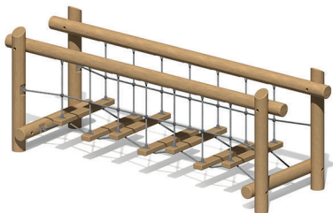
CO-121 Спортивное оборудование "Подвесной мост" Д 3800 / Ш 1250 / В 1400 мм
