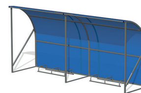
ТН-05 Парковка для колясок Д 5000 / Ш 1405 / В 2400 мм
