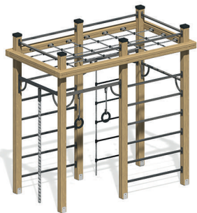
ГК-10 Гимнастический комплекс Д 2540 / Ш 1400 / В 2555 мм
