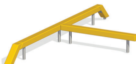
СО-03.7М Спорт. оборудование "Бум-бревно" Д 4310 / Ш 1900 / В 400 мм
